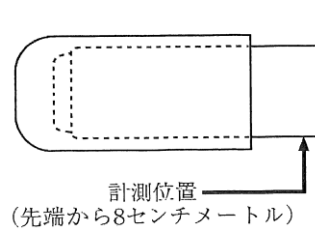
<ちくとうの最小直径値の計測方法>
