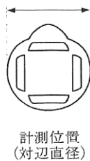
<竹刀の先革長、先端部最小直径値の計測方法>
